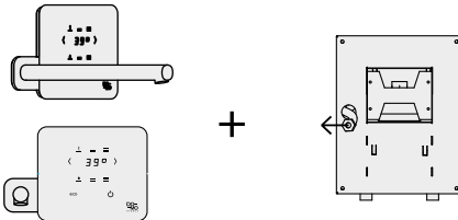
DESIGN PIASTRA DI FISSAGGIO IN ACCIAIO INOX VISTA LATERALE E FRONTALE STAINLESS STEEL FIXING PLATE DESIGN LATERAL AND FRONT VIEW
