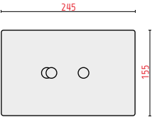
PLACCA WC IN ACCIAIO INOX A DOPPIO FLUSSO STAINLESS STEEL DUAL FLUSH WC PLATE
