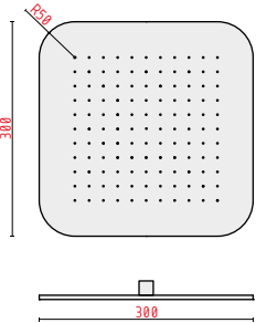
SOFFIONE 300X300 mm HEAD SHOWER 300X300 mm
