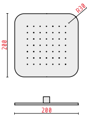
SOFFIONE 200X200 mm HEAD SHOWER 200X200 mm
