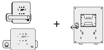
DESIGN PIASTRA DI FISSAGGIO IN ACCIAIO INOX VISTA LATERALE E FRONTALE STAINLESS STEEL FIXING PLATE DESIGN LATERAL AND FRONT VIEW
