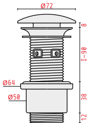
PILETTA PER LAVABO/BIDET WASTE DRAIN FOR WASHBASIN/BIDET ACCIAIO INOX: SATINATO – LUCIDO STAINLESS STEEL: SATIN – CHROME
