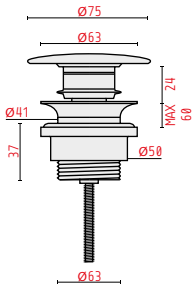
PILETTA PER LAVABO/BIDET WASTE DRAIN FOR WASHBASIN/BIDET CERAMICA BIANCA WHITE CERAMIC
